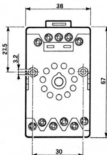
ZVU (11-pin)
