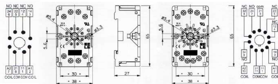
ZVE8 (8-pin)
