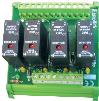
ET-MSZ04 4 Way
