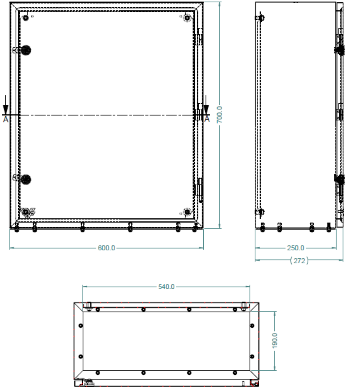
SECTION A-A SCALE 1 : 5
