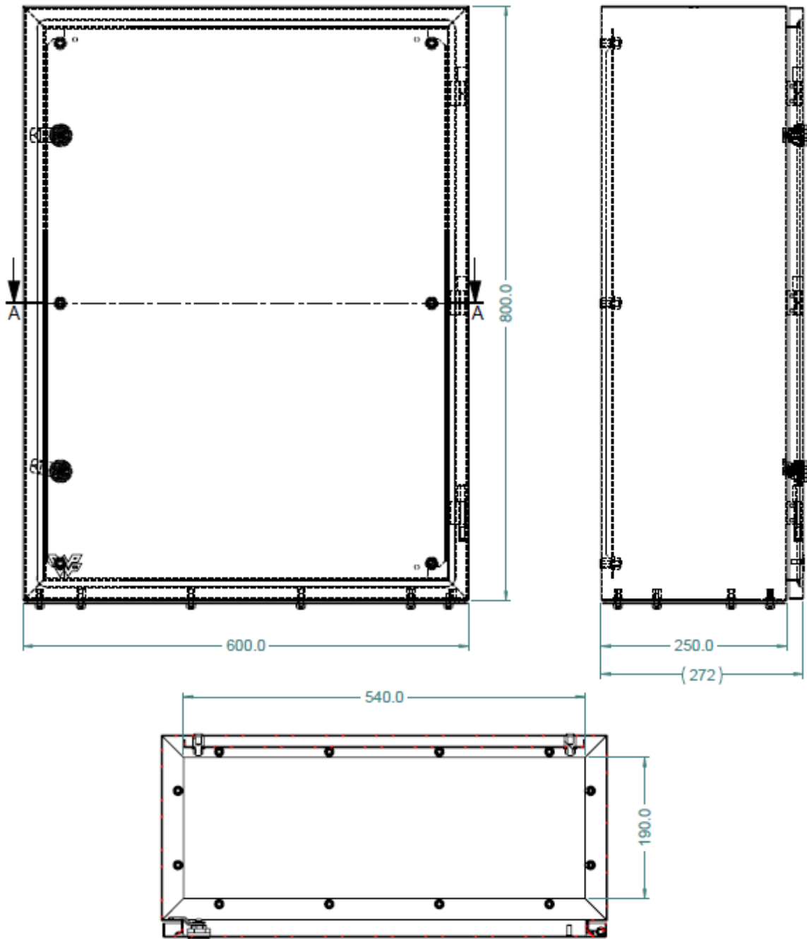
SECTION A-A SCALE 1 : 5
