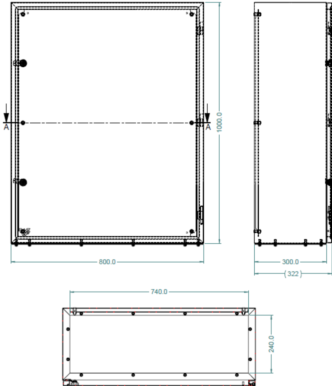
SECTION A-A SCALE 1 : 6.5
