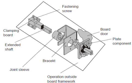
1000~1600A handle
